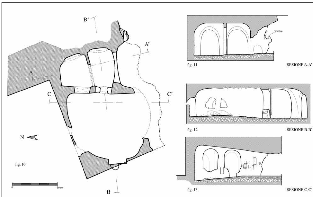
fig. 10 Chiesa del Crocifisso a Chiancalata – Pianta, con indicazione di sezioni.
